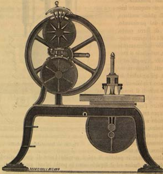
Fig. 32. — Apparecchio Domasin di Ficarolo (Rovigo) Erectator, per sciogliere il lievito, impastare la farina, e ridurla per la lavorazione meccanica.
